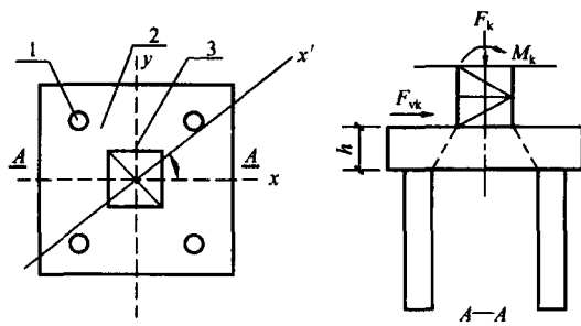
图 3.2.4 塔式起重机方形承台桩基础
