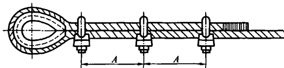
图 6.2.4 钢丝绳夹压板布置图
