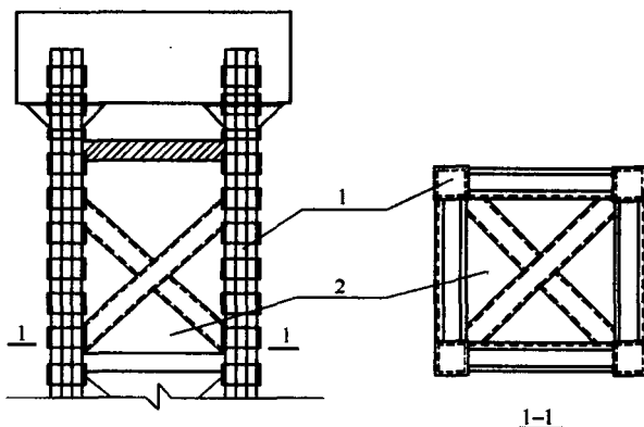
图 3.2.5 塔式起重机组式基础的钢格构柱示意
