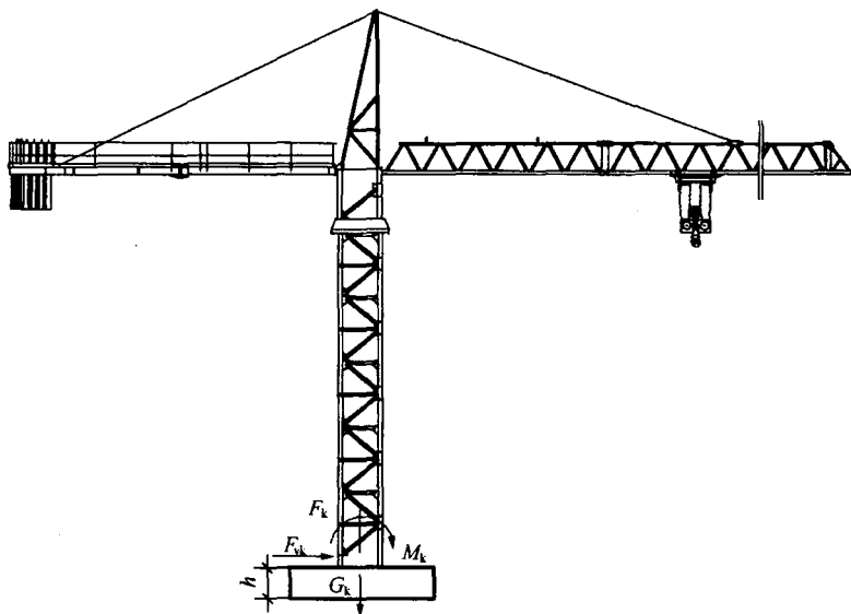
图 3.2.3 塔式起重机板式基础计算简图
