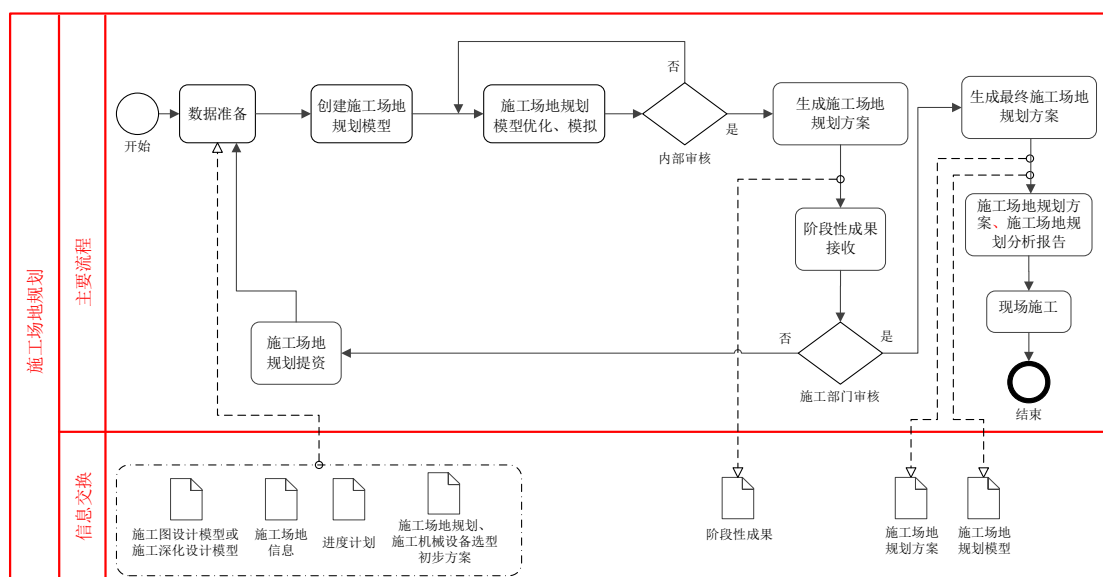
图 6.1.3 施工场地规划 BIM 应用操作流程
