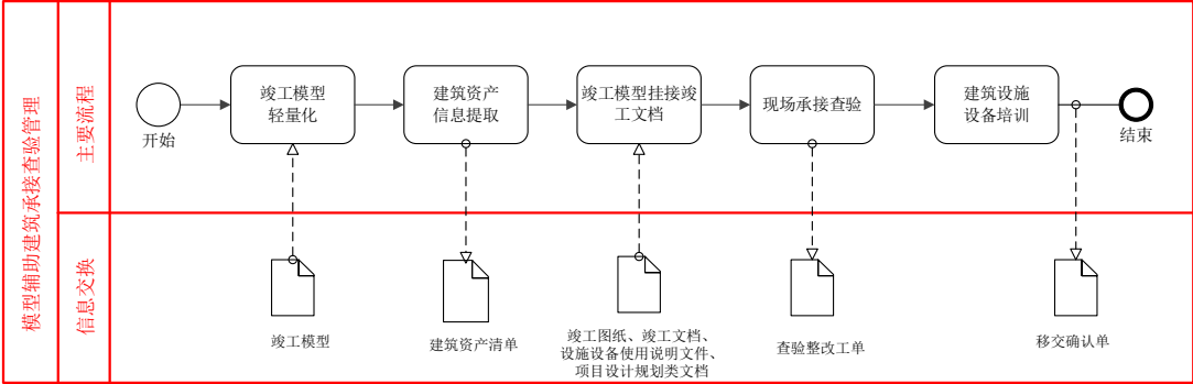
图 8.8.3 模型辅助建筑承接查验管理 BIM 应用操作流程
