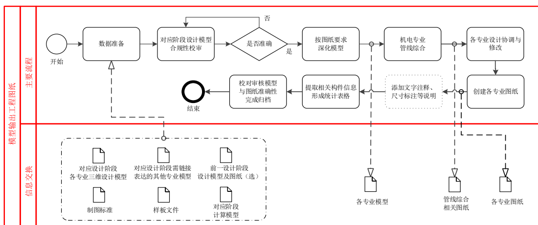
5.5.3 模型输出工程图纸 BIM 应用操作流程
