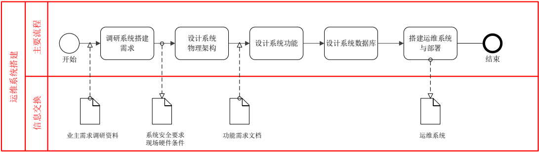
图 9.3.3 运维系统搭建 BIM 应用操作流程图
