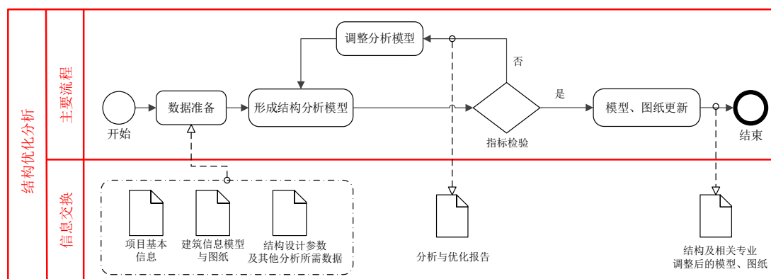
图 4.4.3 结构优化分析 BIM 应用操作流程
