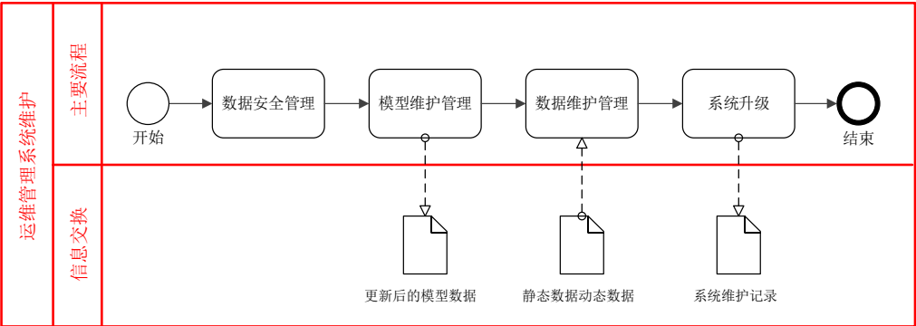
图 9.4.3 运维管理系统维护 BIM 应用操作流程图
