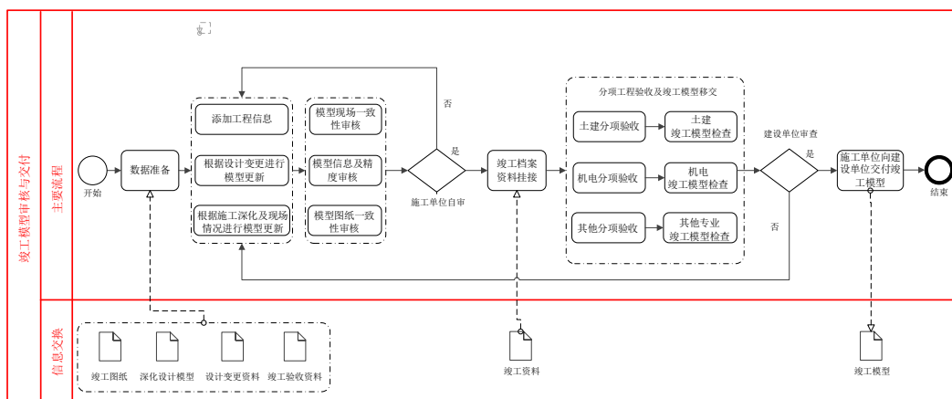
图 8.7.3 竣工模型审核与交付 BIM 应用操作流程图
