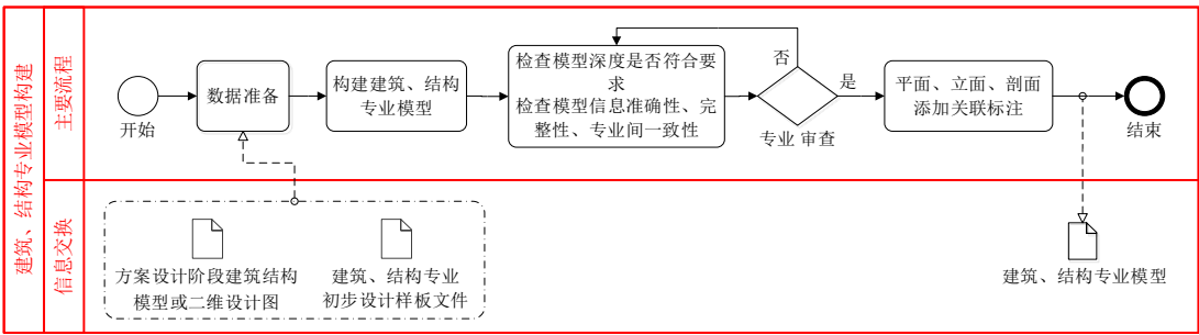
图 4.1.3 建筑、结构专业模型构建 BIM 应用操作流程
