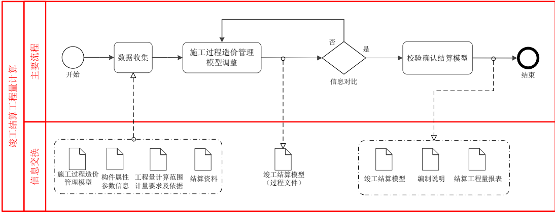
图 8.10.3 竣工结算工程量计算 BIM 应用操作流程
