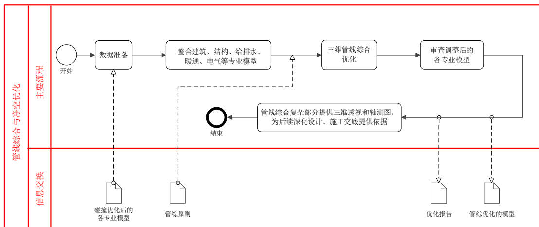
图 5.4.3 管线综合与净空优化 BIM 应用操作流程
