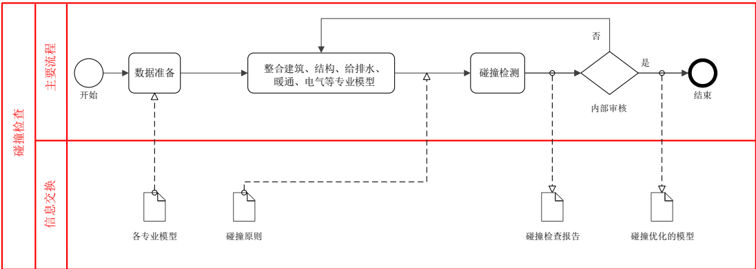
图 5.3.3 碰撞检查 BIM 应用操作流程图
