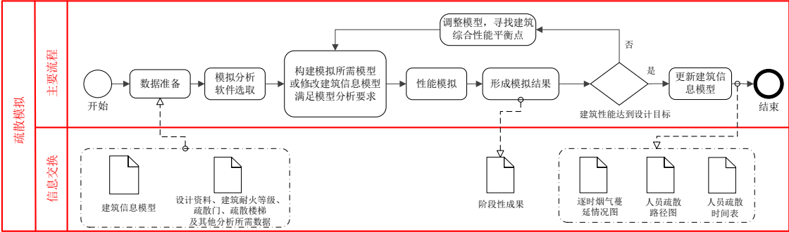
图 4.9.3 疏散模拟 BIM 应用操作流程
