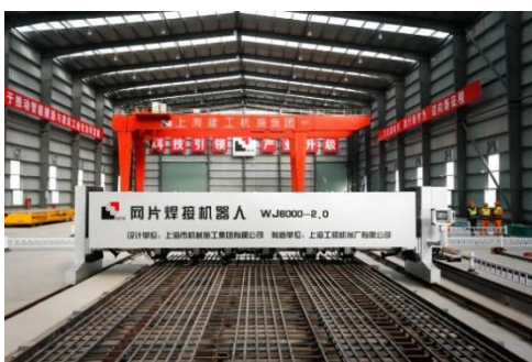
图5.12 地下连续墙钢筋笼焊接机器人
