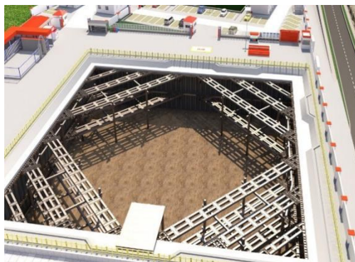
图5.25 围护效果图
