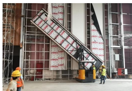
图5.15 超大墙面板块半自动安装机器人
