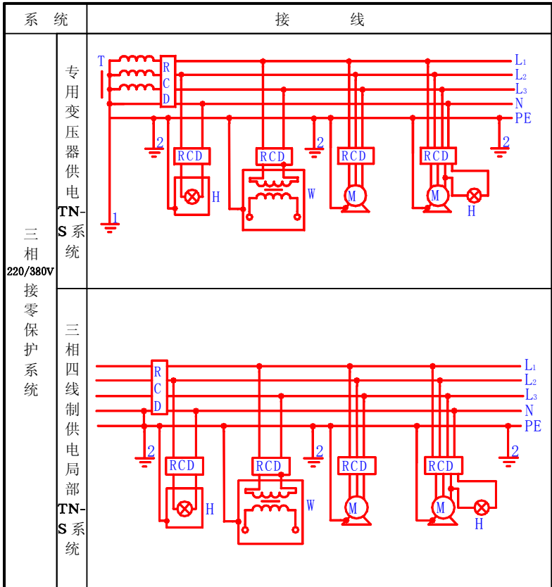
图8.2.14 漏电保护器使用接线方法示意
