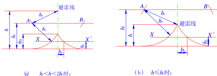
图 B. 0. 2 单根架空避雷线的保护范围
