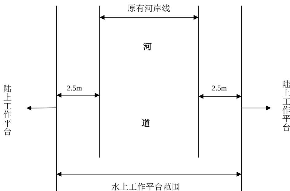
图 3.1.1 水上、陆上工作平台划分图示
