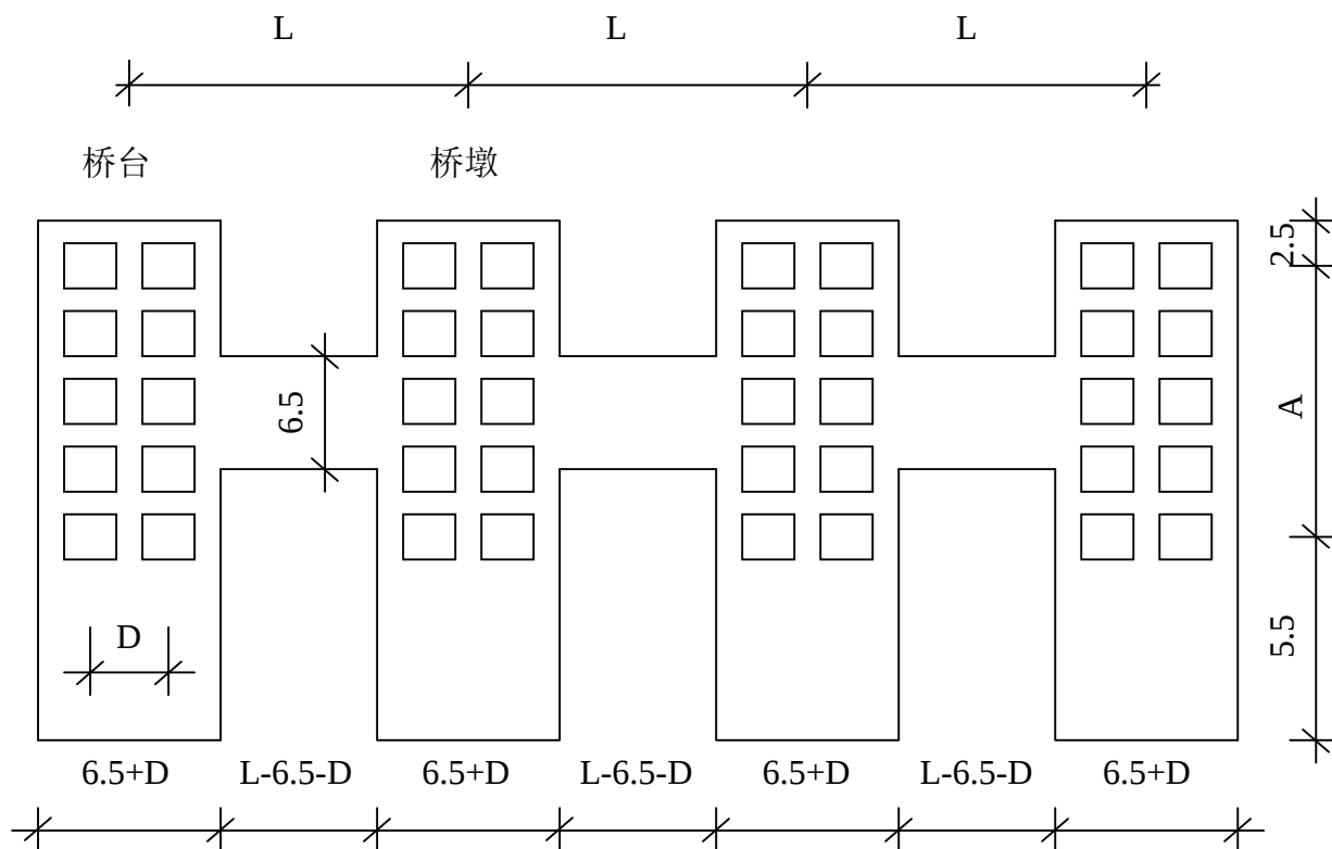
图 3.1.2 工作平台面积计算示意图
