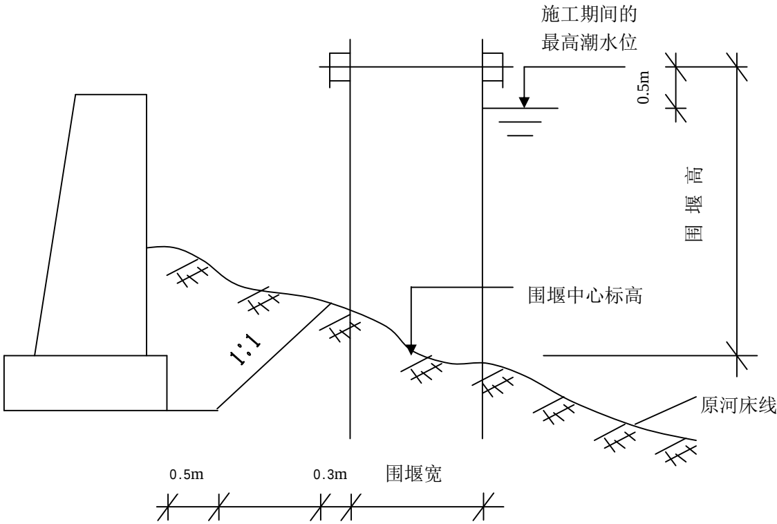
图 7.1.1 围堰高度计算示意图
