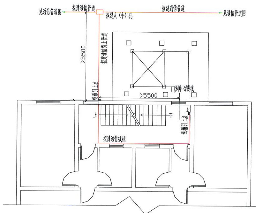
图 1 平层入户型通信管道避让加装电梯位置示意图
