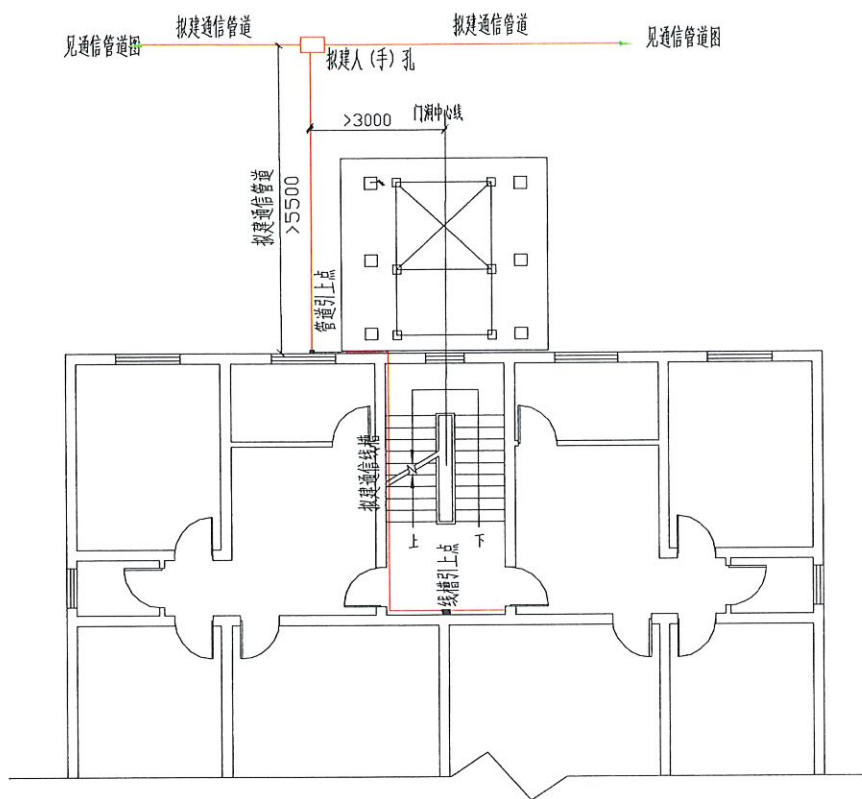
图 2 半平台入户型通信管道避让加装电梯位置示意图
